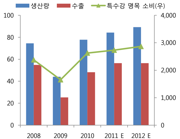
그림 21. 건설기계 국내 생산, 수출 및 특수강 명목소비 (단위:천 대, 억 원)
