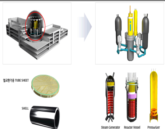
그림 31. 원자력 발전용 단조품
